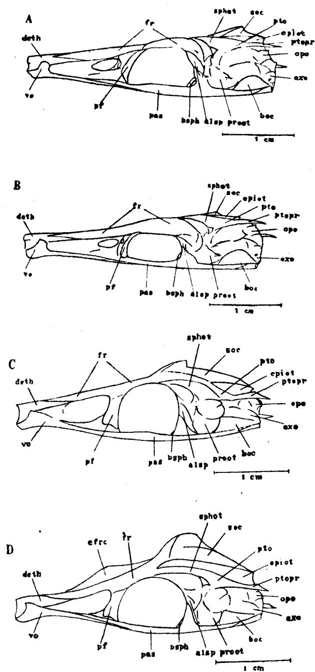
Fig. 13. Neurocranium, lateral view. A. T. lepturus . B. L. savala . C. E. intermedius . D. E. muticus .
