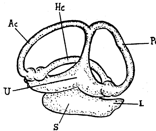
Fig. 28. Membranous labyrinth of T. lepturus (diagrammatic). Ac : Anterior canal; Hc : Horizontal canal; L : Lagena; Pc : Posterior canal; S : Sacculus; U : Utricle.
