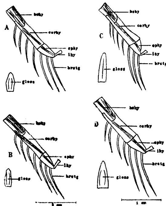
Fig. 18. Hyoid arch and glossohyal. A. T. lepturus . B. L. savala . C. E. intermedius . D. E. muticus .
